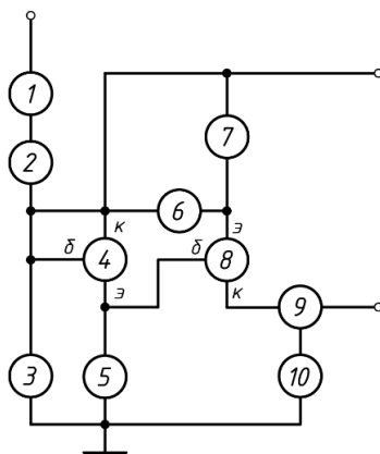
Логический элемент «ИЛИ»
