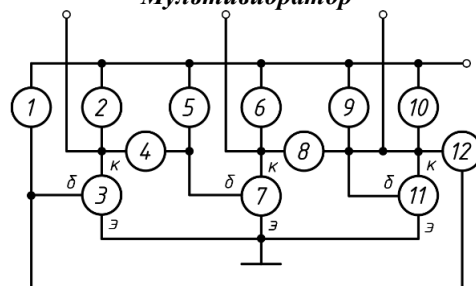
Мультивибратор
