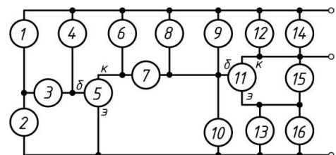
Генератор
