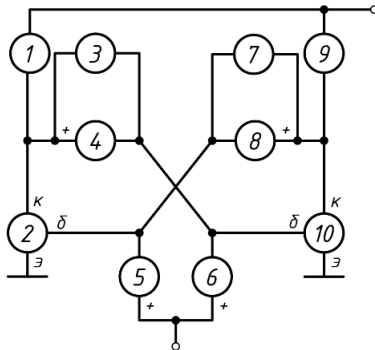
Триггер
