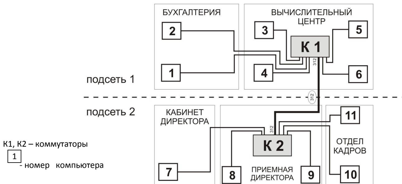
Рисунок 4.1 – Схема локальной сети
