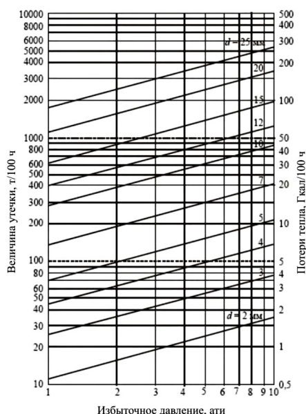
Рис. 1. Номограмма для определения величины
