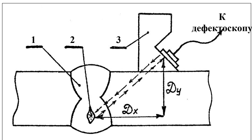
Рис. 3 Схема определения координат дефекта с помощью наклонной касательной головки:
