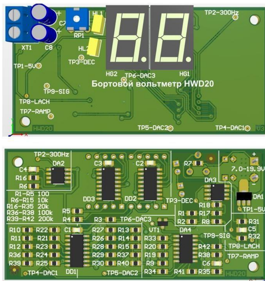
Рисунок 1 - Внешний вид устройства в сборе
