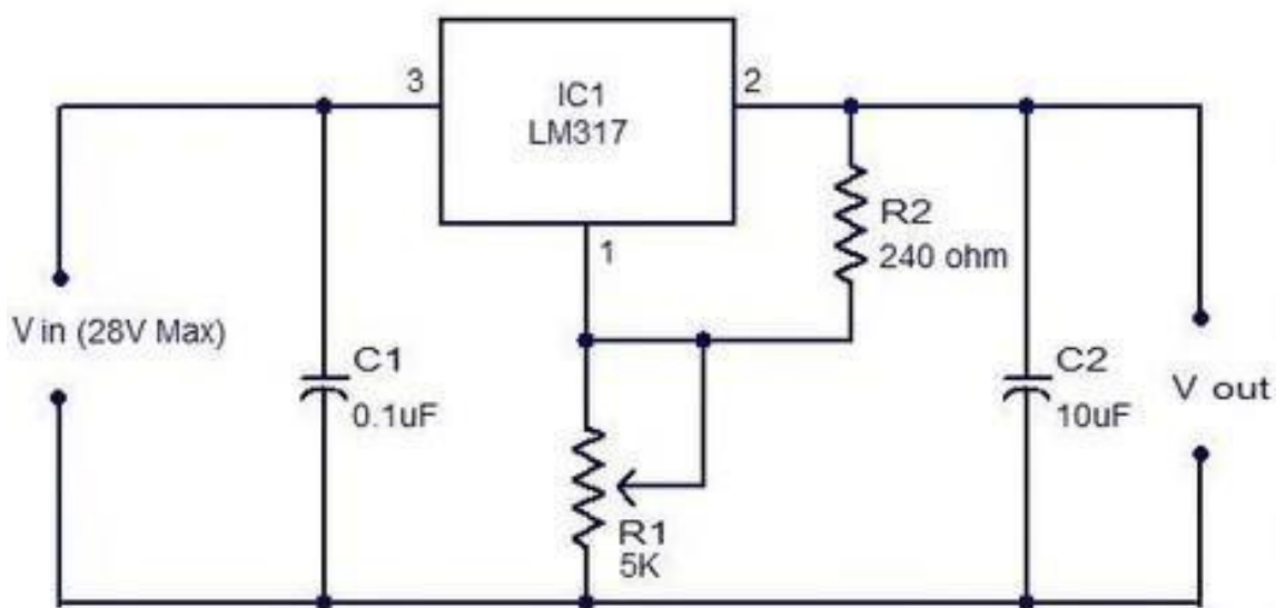
Типовое применение микросхемы в качестве стабилизатора
