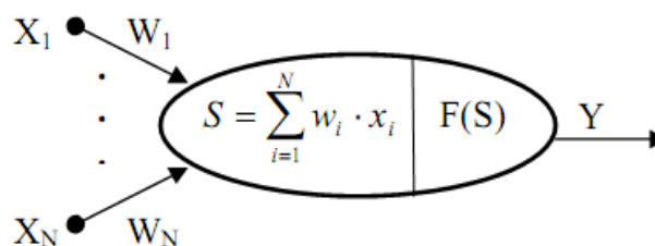
Рис. 4. Формальный нейрон (математическая модель)
