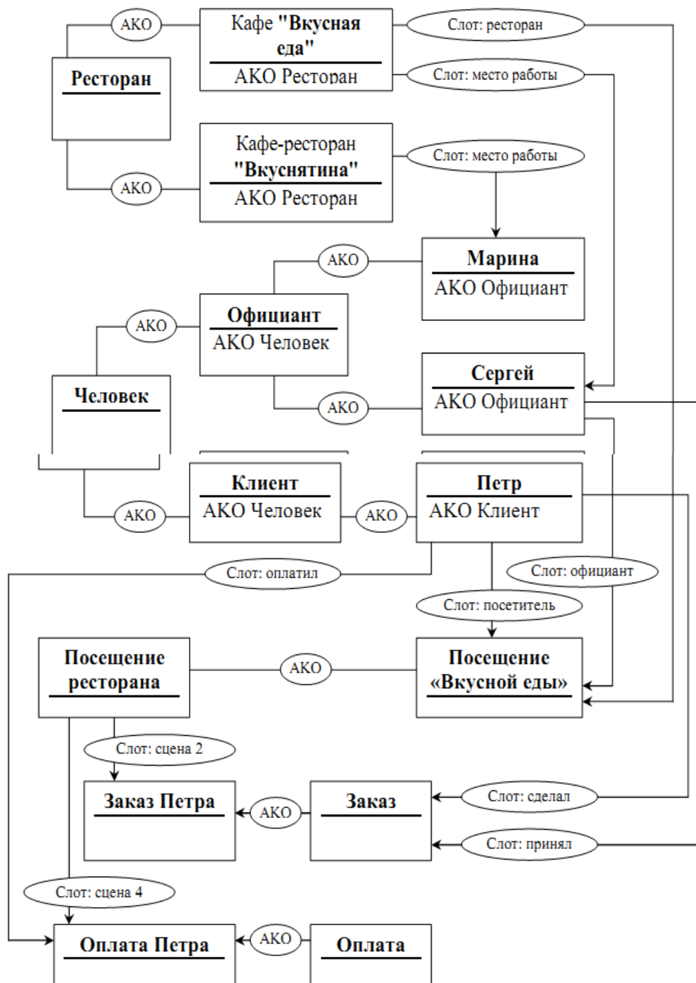
Рис. 3. Схема фреймов для предметной области «Ресторан».
