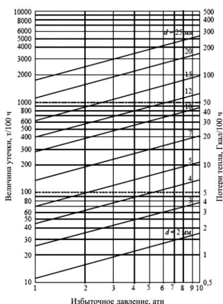
Рис. 1. Номограмма для определения величины утечки сетевой воды и потерь тепла (при T_v = 55 °C).
