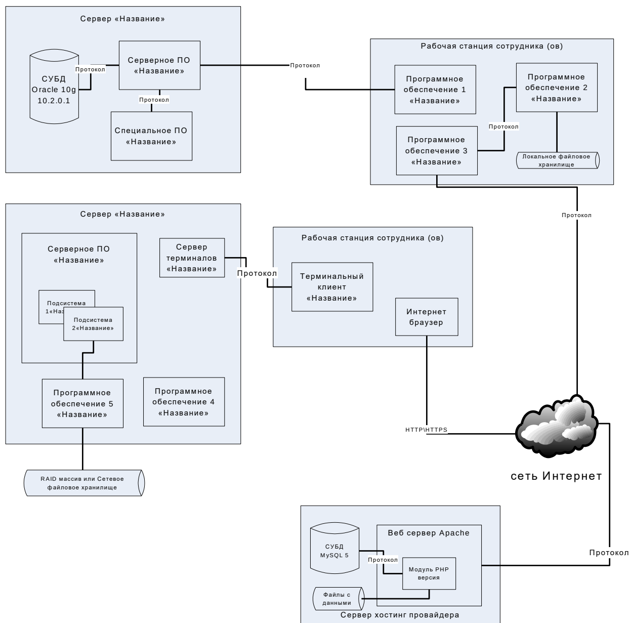
Рис.3. Пример программной архитектуры предприятия
